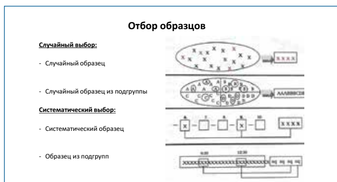
Рис. 7. Способы отбора образцов. Случайный образец – каждая единица имеет одинаковую известную вероятность стать образцом. Случайный образец из подгруппы – количество образцов должно быть пропорционально количеству подгрупп. Систематический образец – отбор каждого N-го образца (например, каждого 3-го). Образец из подгрупп – отбор N-го количества единиц за единицу времени (формирование среднего образца из подгруппы)
