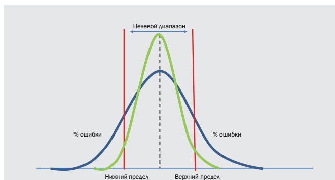
Рис. 3. Пример нормального распределения
